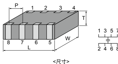
<尺寸>
