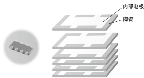
< 结构示例 >
