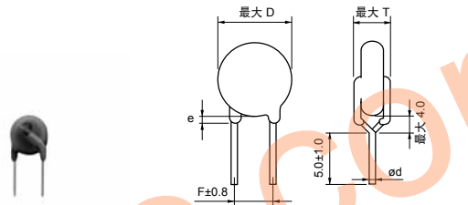
【散装】 垂直有弯头短型（B5）
